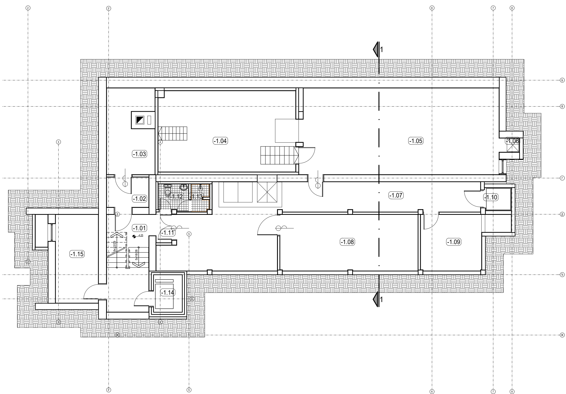
ОСНОВА ПОДА ПОДРУМА, Р 1:100
