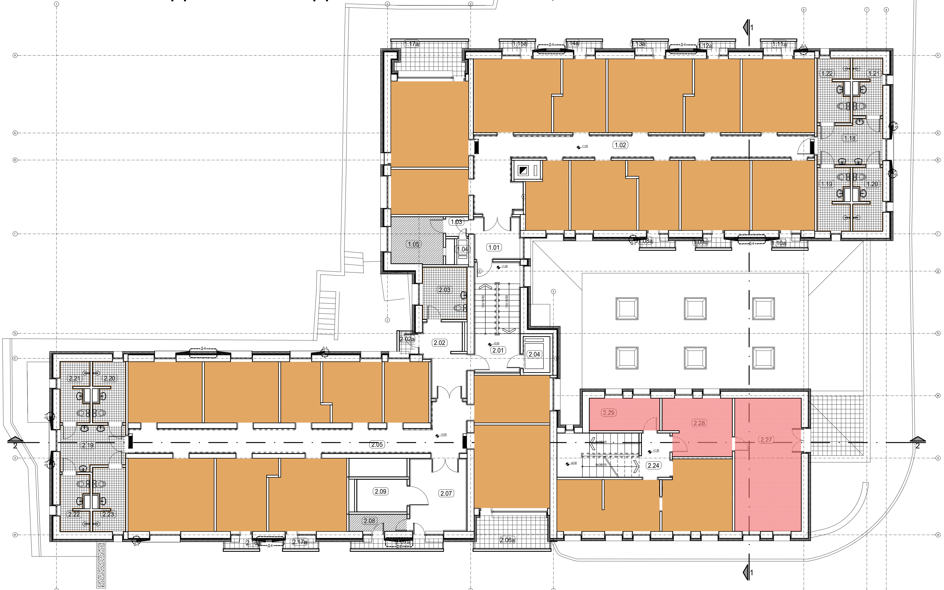
ОСНОВА ПОДА ТРЕЋЕГ И ЧЕТВРТОГ ПОЛУНИВОА, Р 1:100
